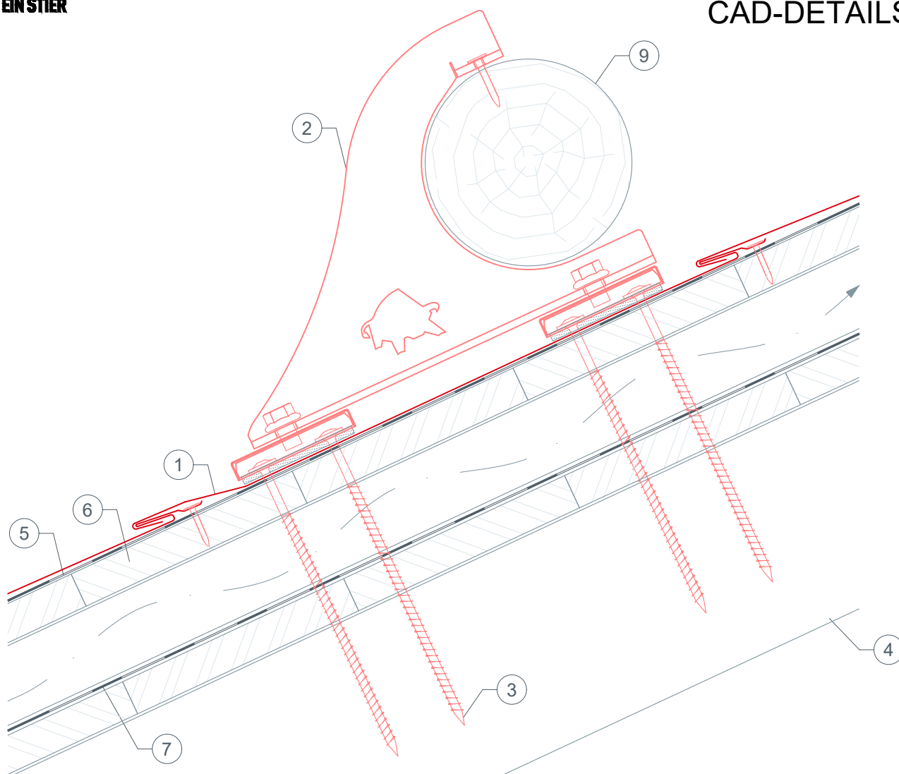
Montage mit Unterlagsplatte
