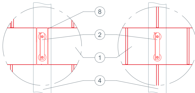
Montage mit Unterlagsplatte
