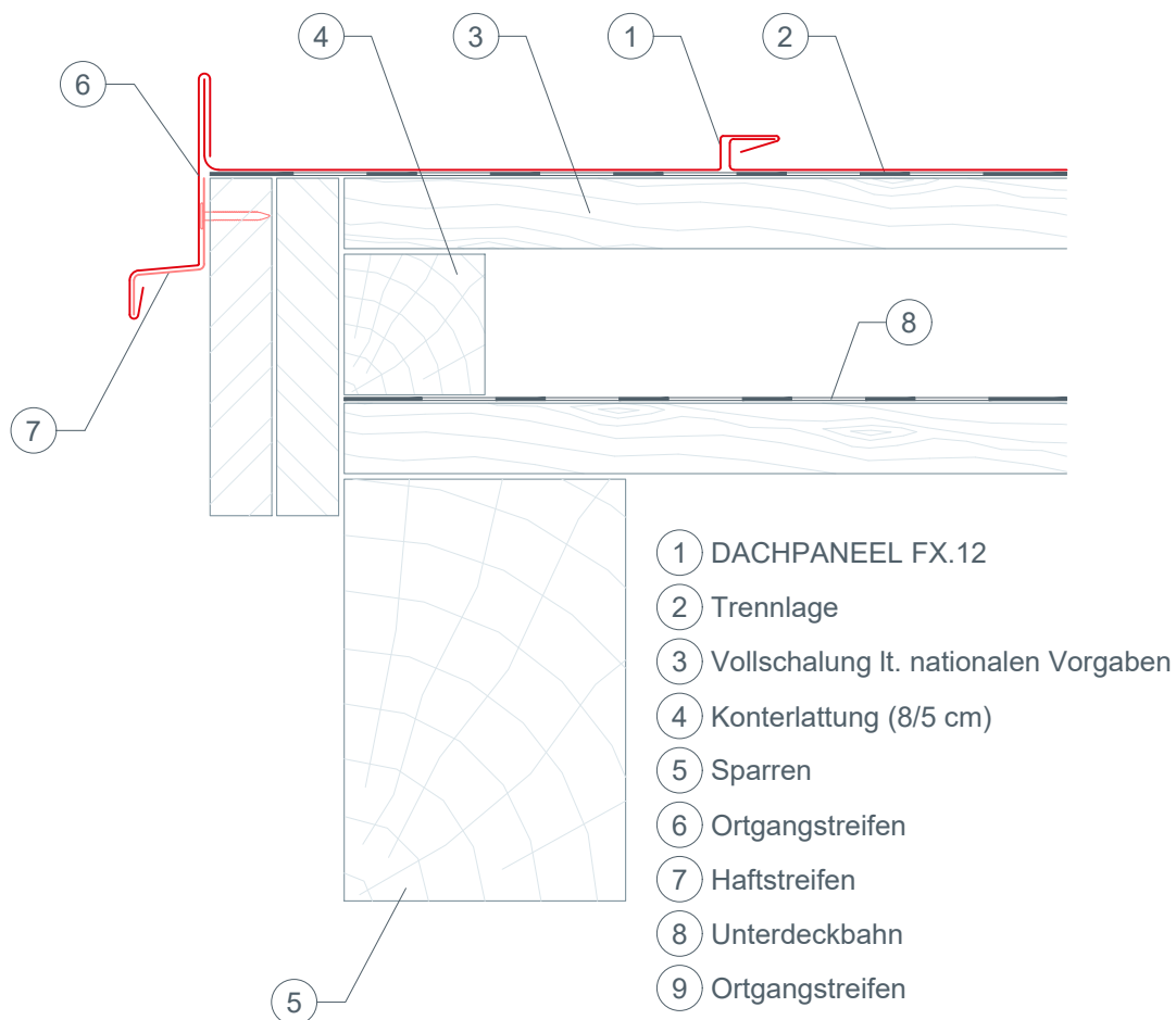
Anschlussvariante
