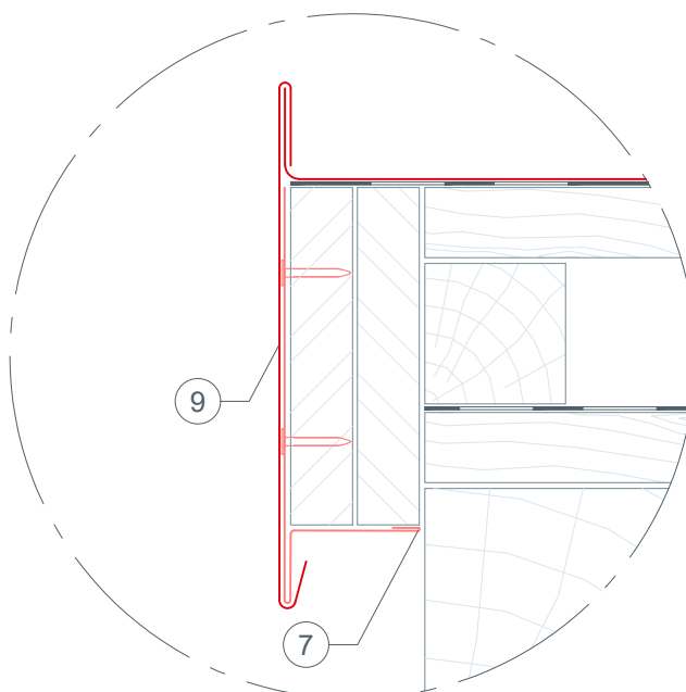
Anschlussvariante
